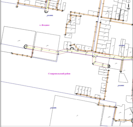
Схема расположения границ публичного сервитута для эксплуатации объекта электросетевого хозяйства
